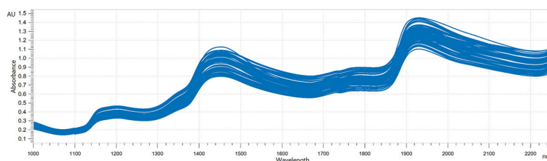
Figure 1. Espectros de infrarrojo cercano de muestras de manzana analizadas en modo de reflexión en un analizador NIR de Metrohm.
