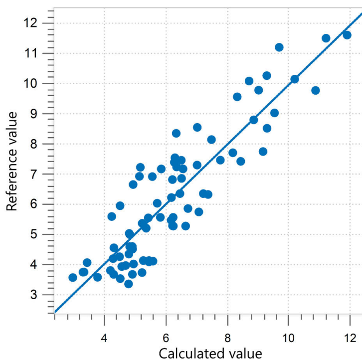
Figure 2. Diagrama de correlación y los respectivos indicadores de rendimiento para la predicción de la firmeza en manzanas con un espectrómetro NIR Metrohm. Los puntos azules representan el conjunto de datos de calibración. En este ejemplo no se utilizó ningún conjunto de validación.
