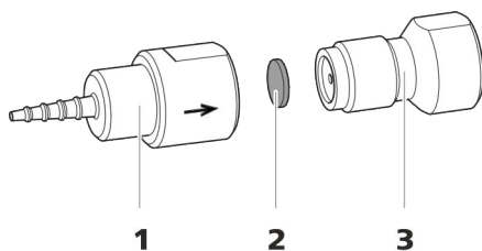
Figura 10 Conexión de tubo de bomba – Sustituir el filtro
