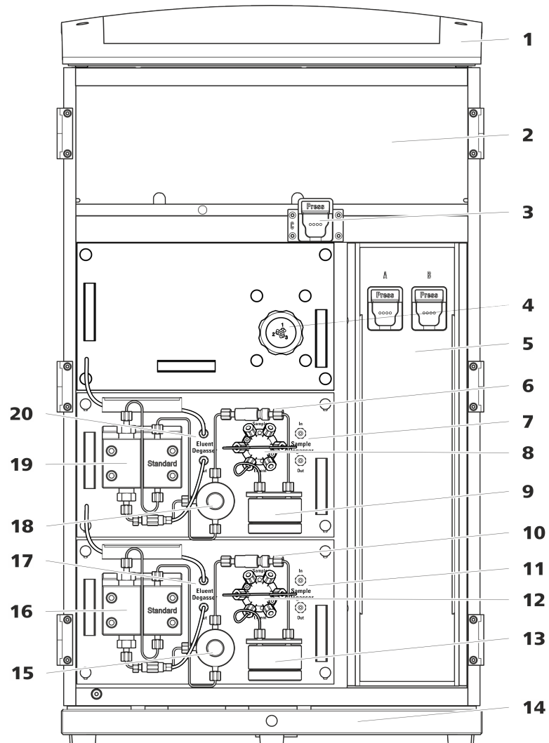
Figure 1 Face avant
