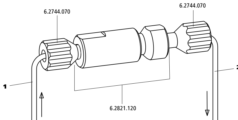
Figura 10 Filtro inline
