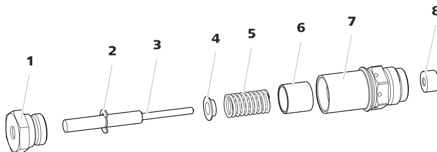
図23 ピストンカートリッジの構成部品
