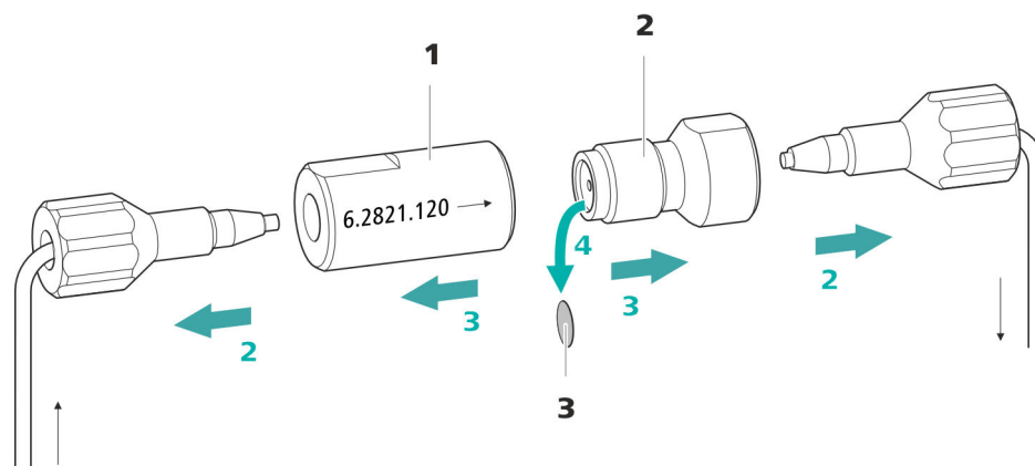
図24 インラインフィルター- フィルターの取り外し
