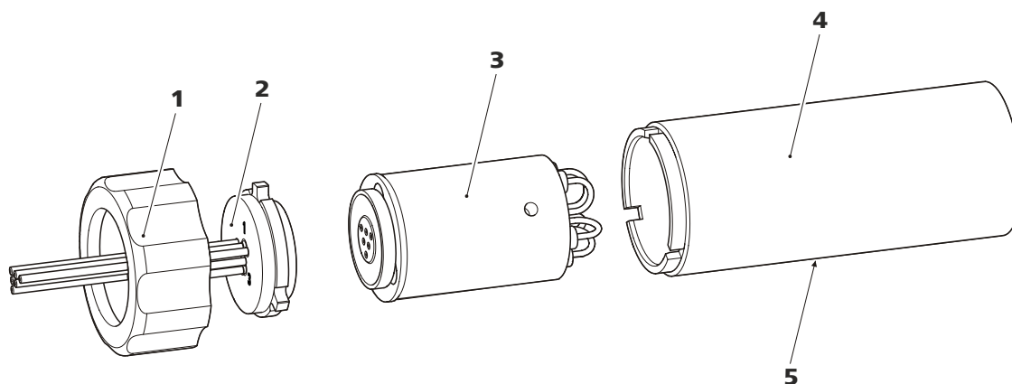
図 25 Metrohm Suppressor Module (MSM) の構成部品
