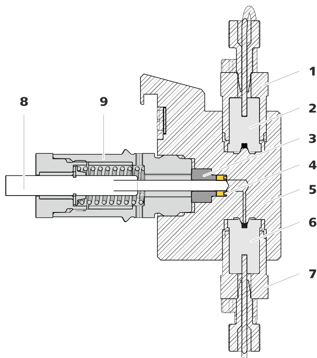
図19 高圧ポンプ- 断面図
