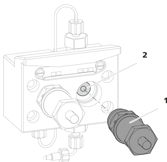
図21 ポンプヘッド- ピストンカートリッジの取り外し
