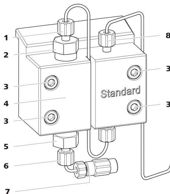
図18 高圧ポンプ- 部品
