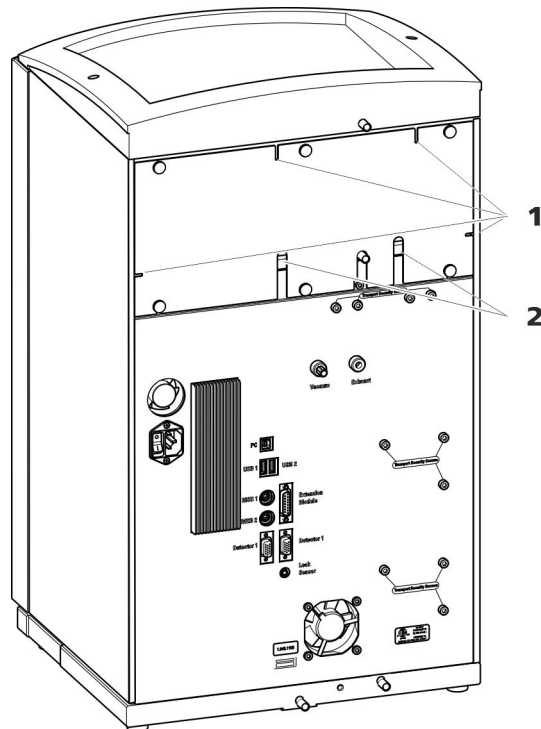
图4 毛细管和电缆的出口
