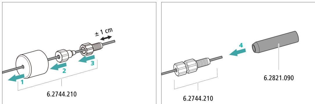
图8 安装加重管和吸液过滤头
