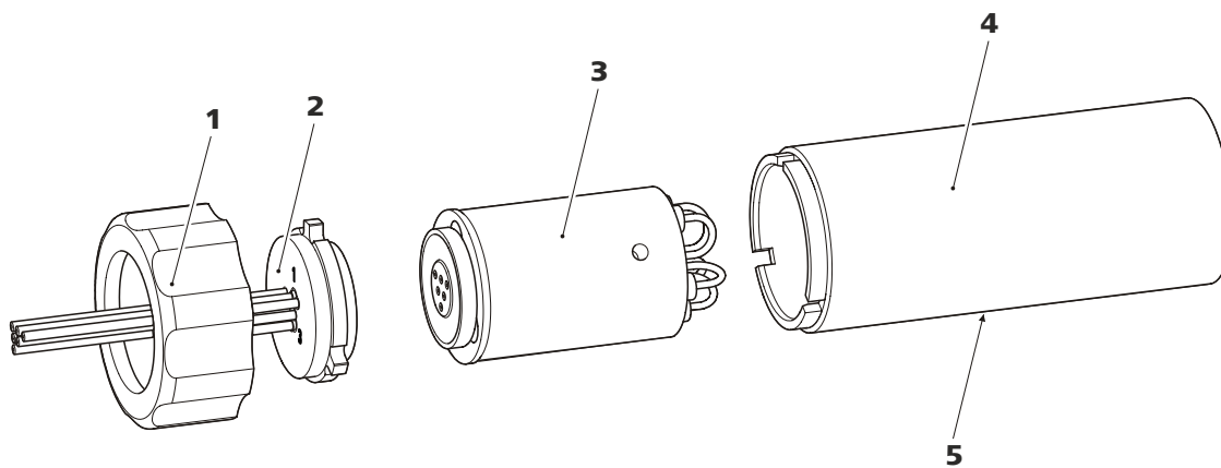
图 21 Metrohm Suppressor Module (万通抑制模块 MSM) 的部件
