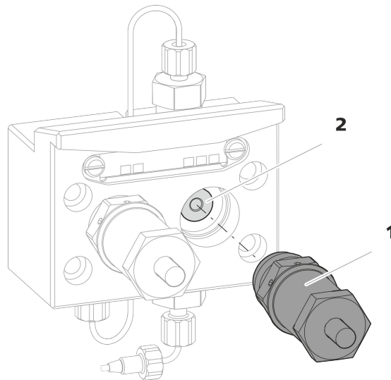
Figure 16 Tête de pompe – retirer la cartouche de piston
